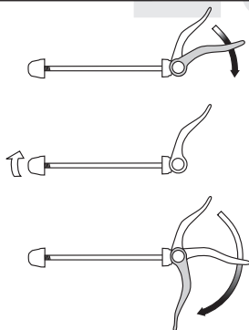
Einstellmutter lockern
